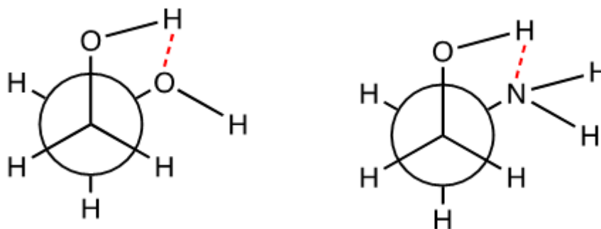
Exemple de conformations éclipsées stabilisées
