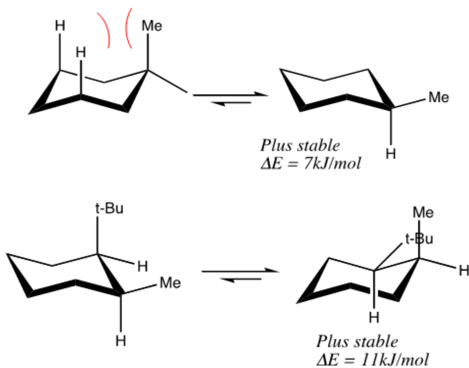
Position axiale vs position équatoriale
