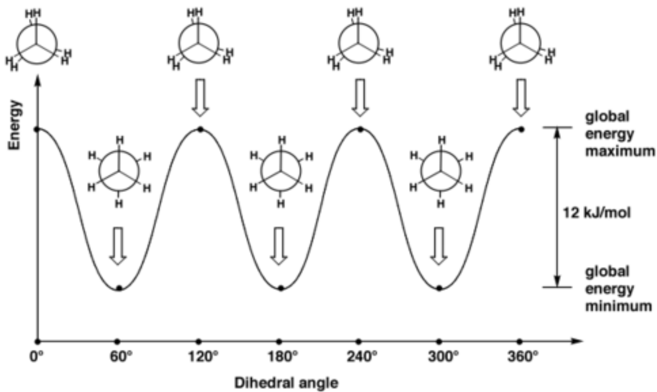
Conformations de l'éthane
