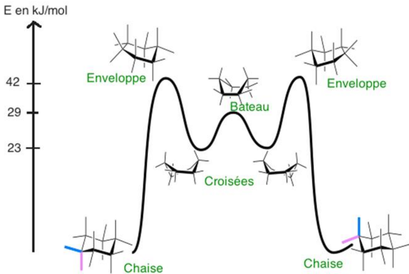
Conformations du cyclohexane
